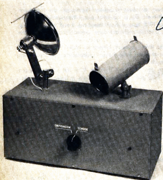
LUXA-VOX zend/ontvanger. Links boven de schijnwerper om te stralen en rechts de ontvangkoker waarin de lghg. Met de knop wordt omgeschakeld van zenden op ontvangen.
